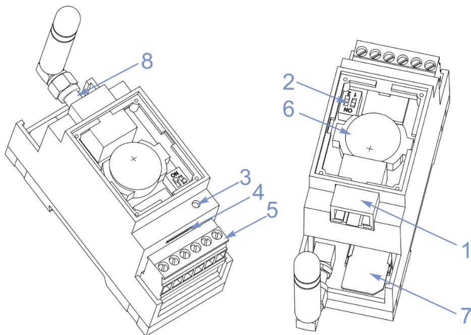
Рисунок 1.5 - Устройство модуля PL307
