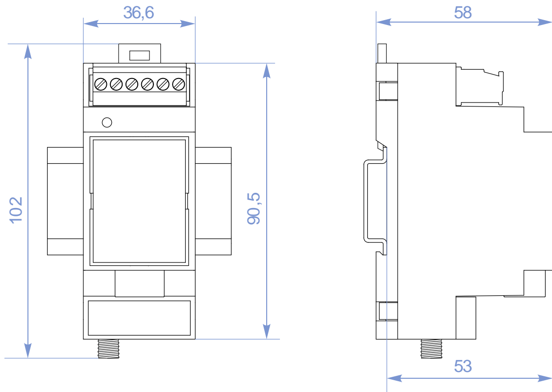
Рисунок 1.2 - Габаритные размеры
