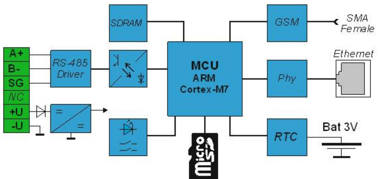
Рисунок 1.3 - Структурная схема
